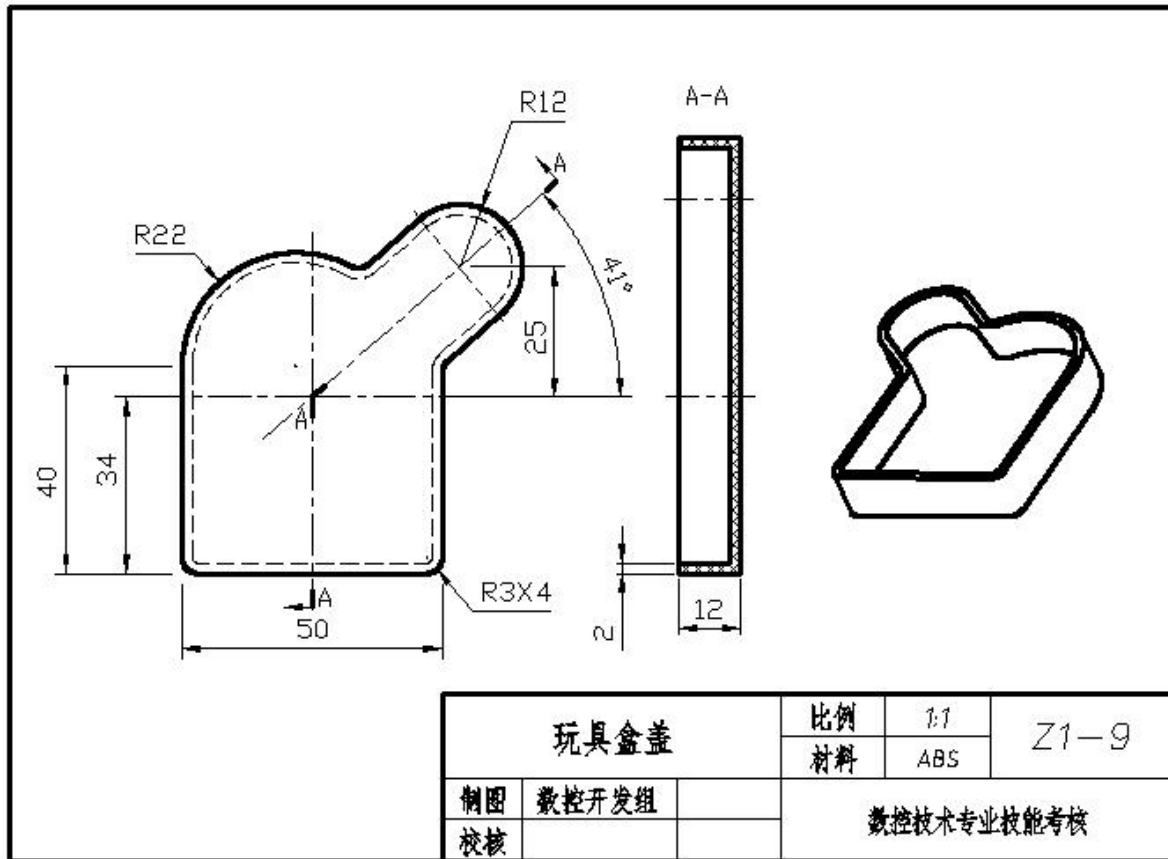
图Z1-9 玩具盒盖
