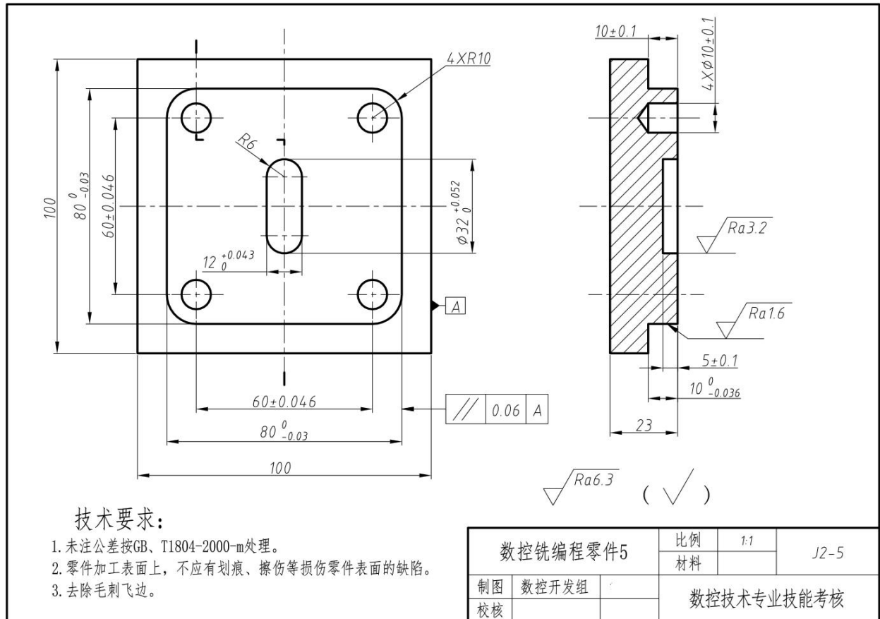
图J2-5 数控铣编程零件5
