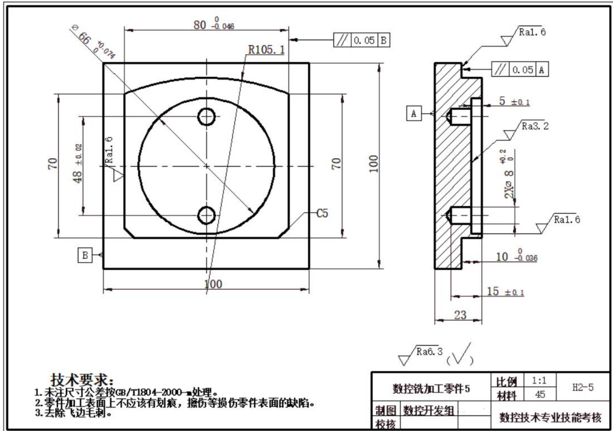
图H2-5 数控铣加工零件5
