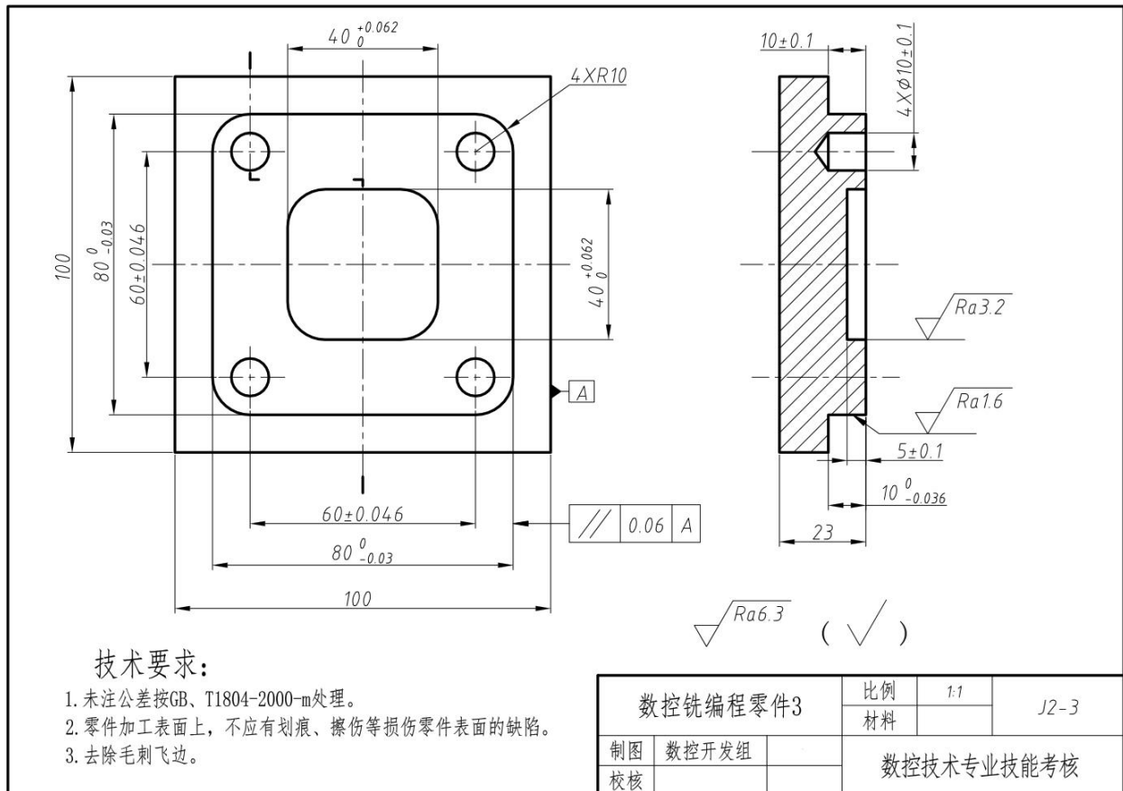
图J2-3 数控铣编程零件3
