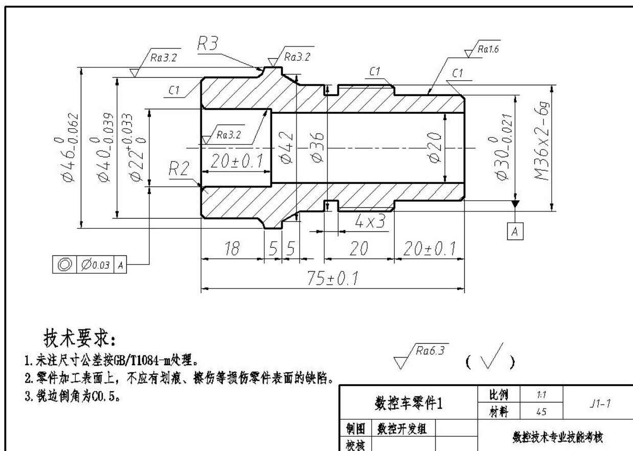
图 J1-1 数控车零件1
