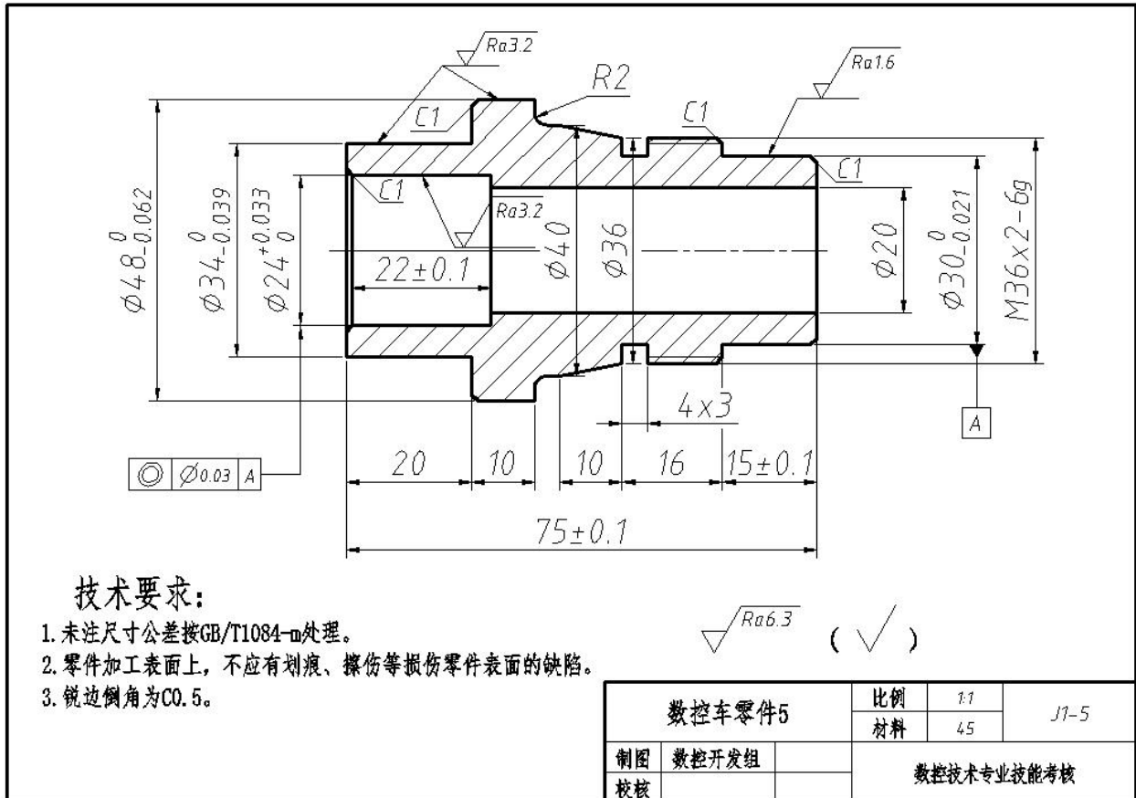
图J1-5 数控车零件5
