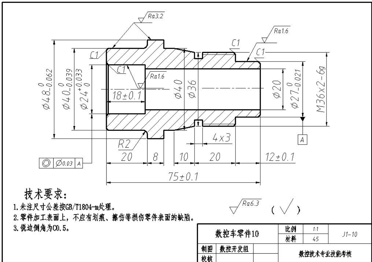
图J1-10 数控车零件10
