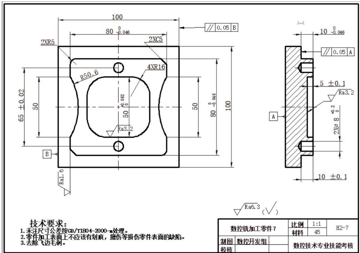
图H2-7 数控铣加工零件7
