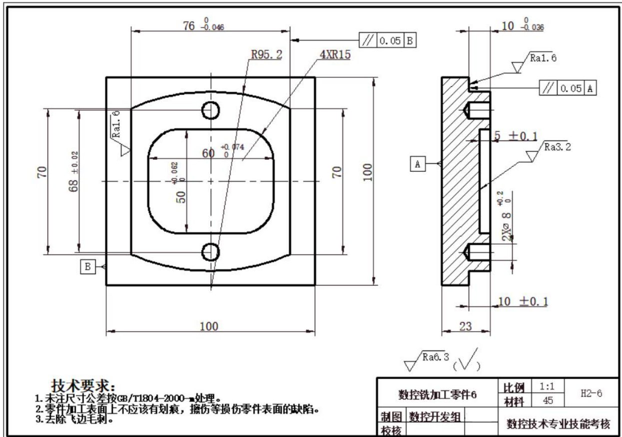
图H2-6 数控铣加工零件6
