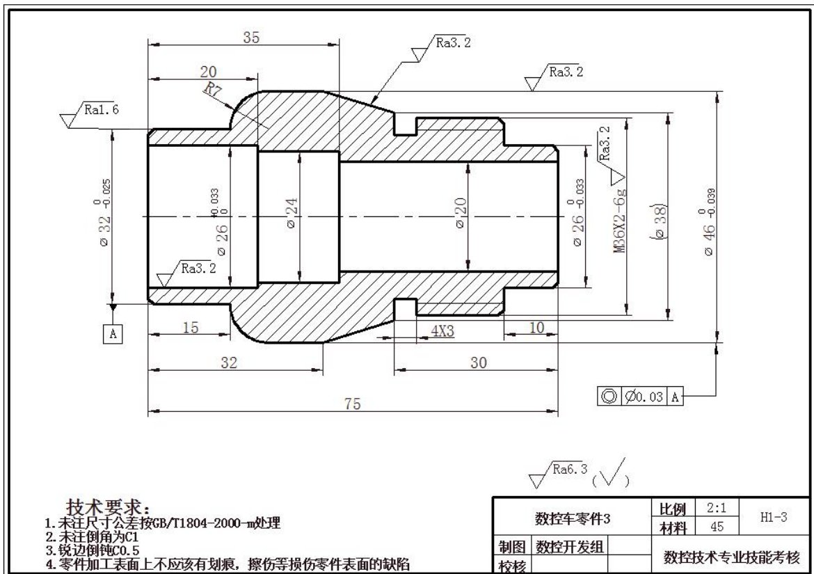
图H1-3 数控车零件3
