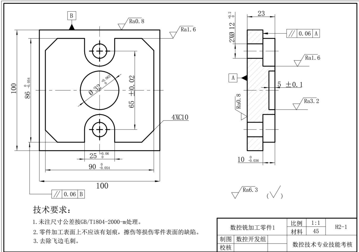
图H2-1 数控铣加工零件1
