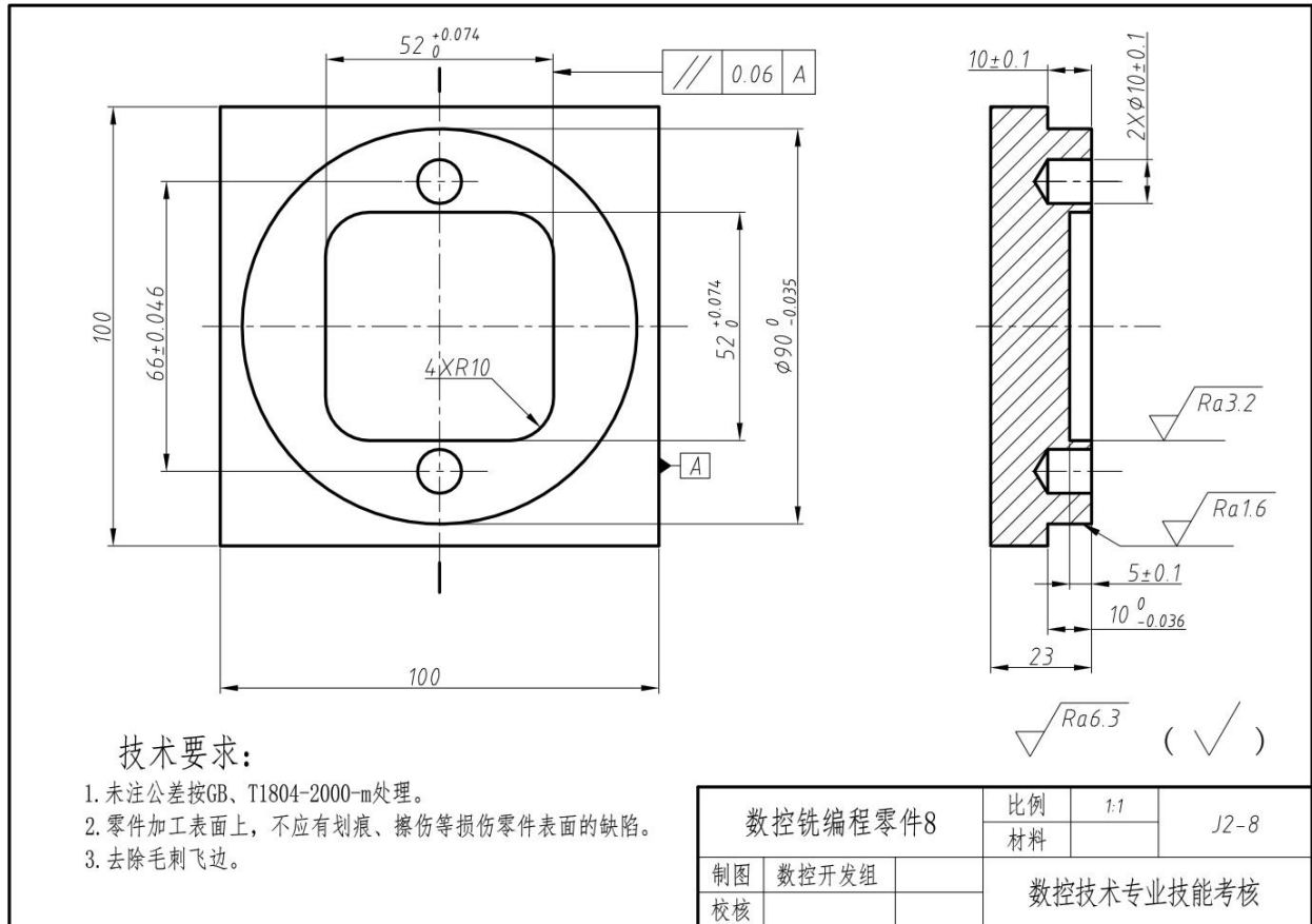
图J2-8 数控铣编程零件8
