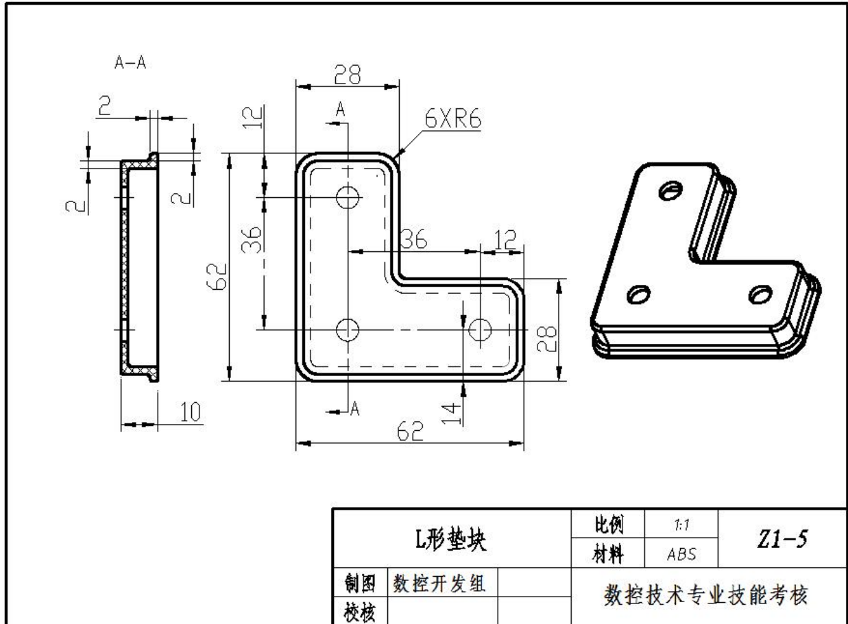
图Z1-5 L形垫块
