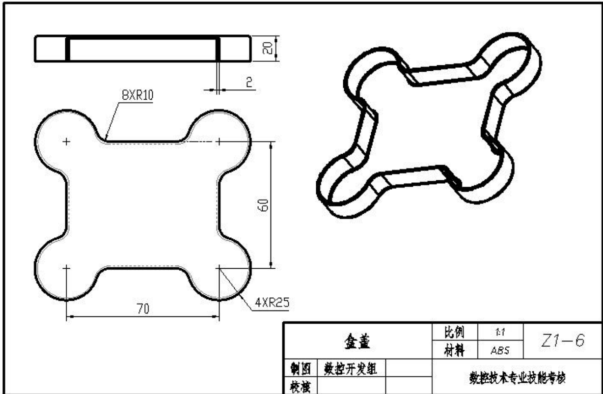
图Z1-6 盒盖
