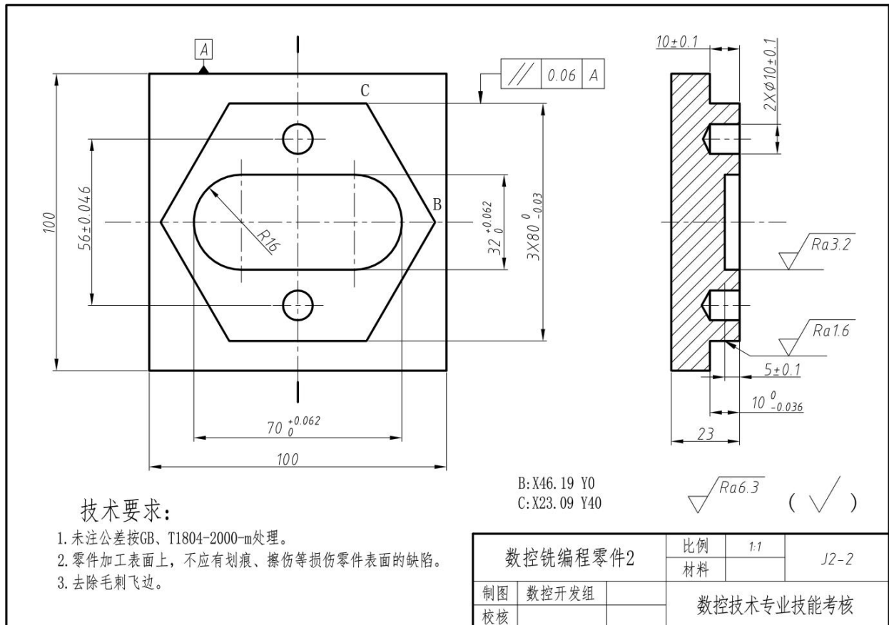
图J2-2 数控铣编程零件2
