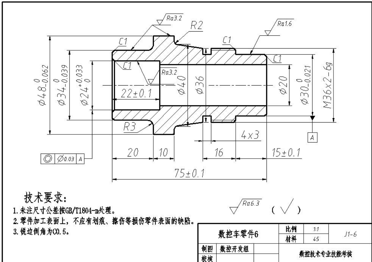
图J1-6 数控车零件6
