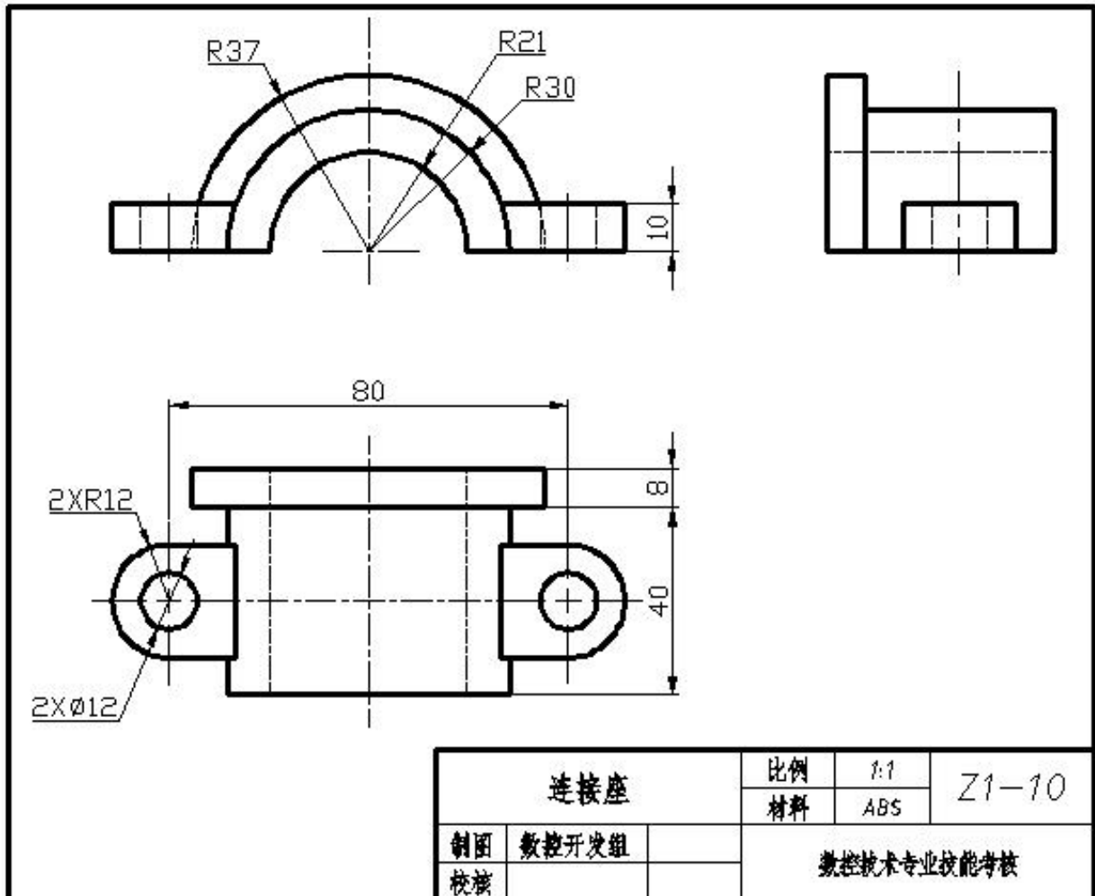
图Z1-10 连接座
