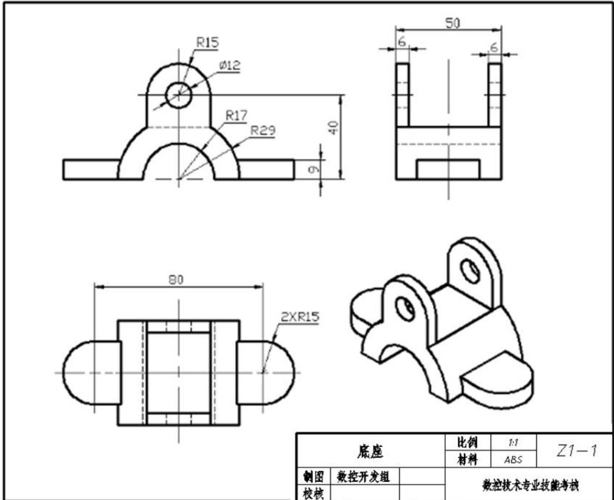
图Z1-1 底座
