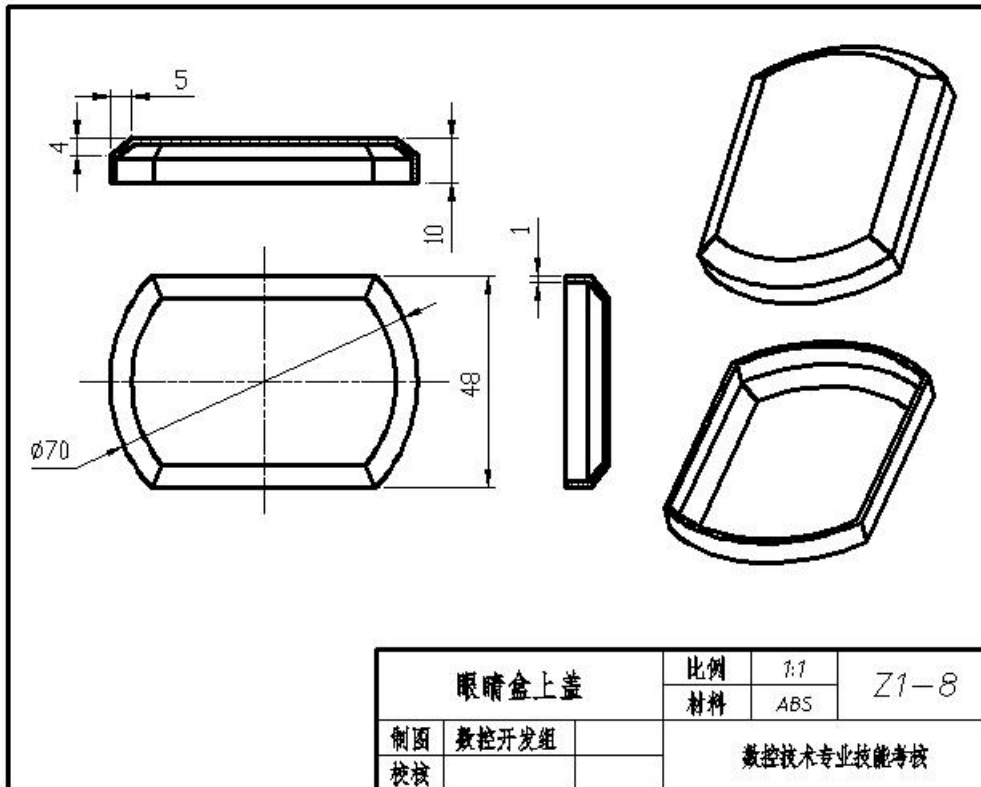
图Z1-8 眼镜盒上盖
