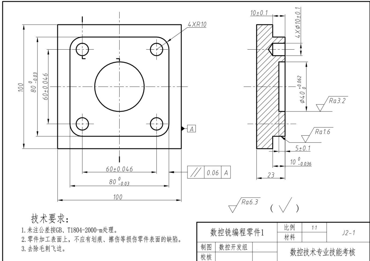
图J2-1 数控铣编程零件1
