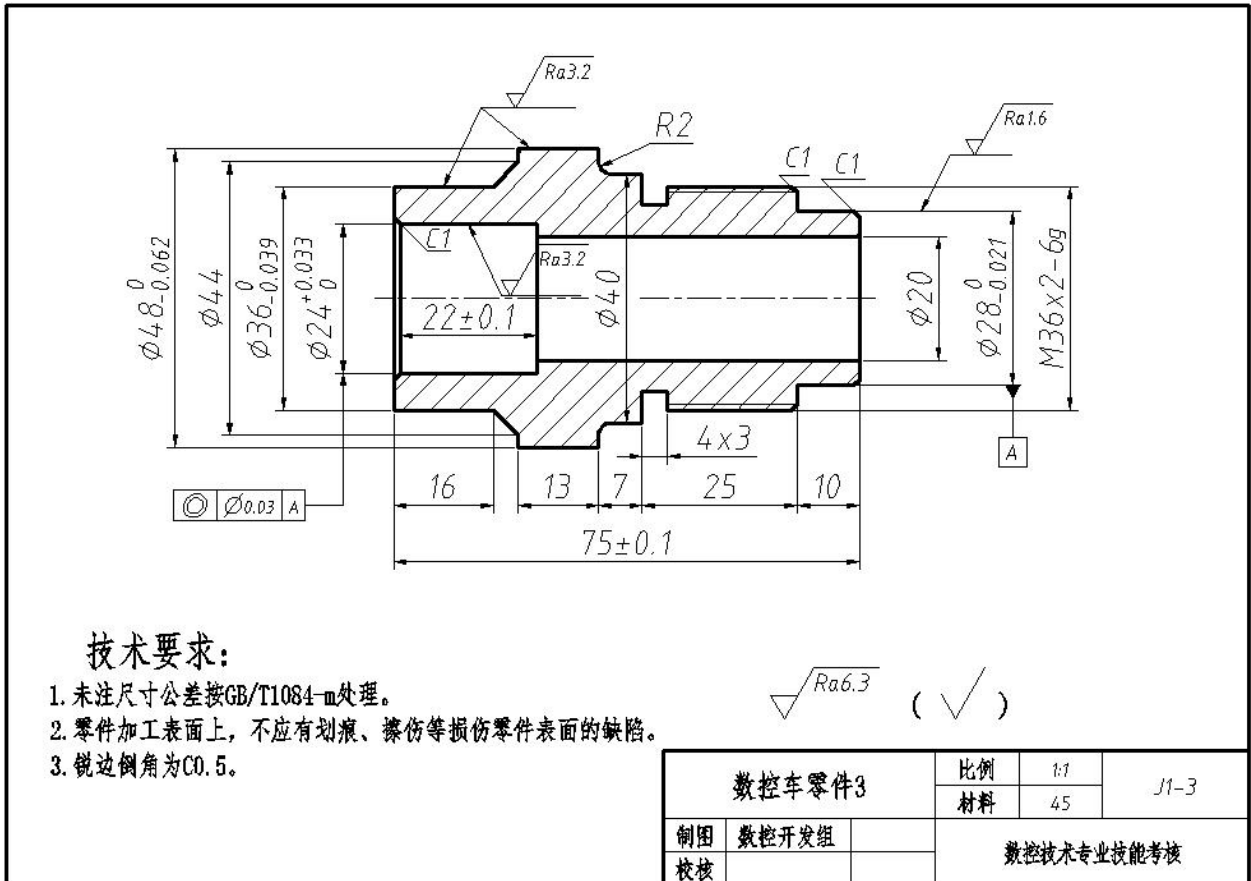
图J1-3 数控车零件3
