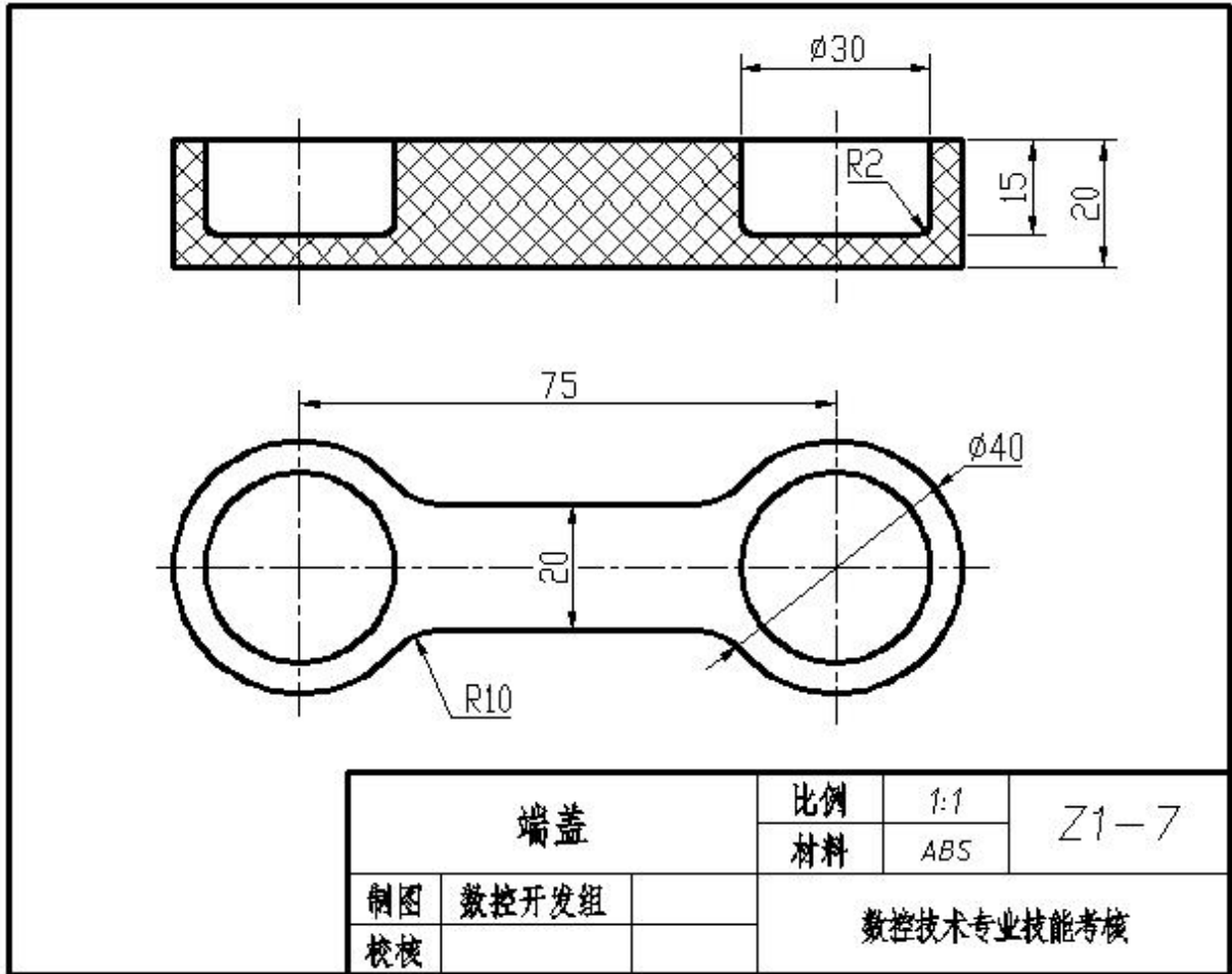
图Z1-7 端盖
