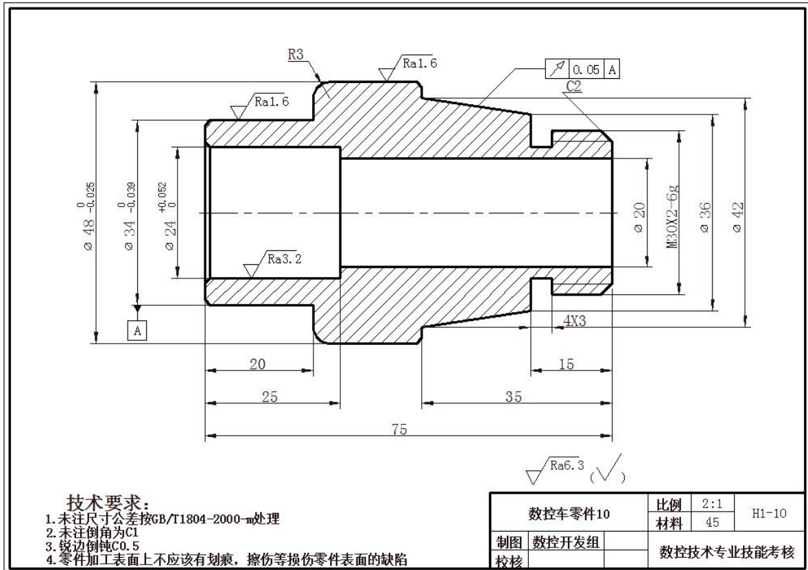
图H1-10：数控车零件10
