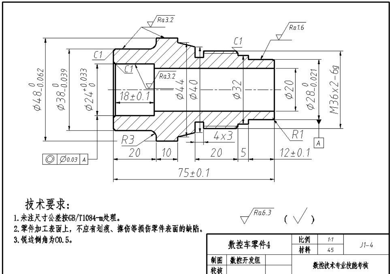
图J1-4 数控车零件4
