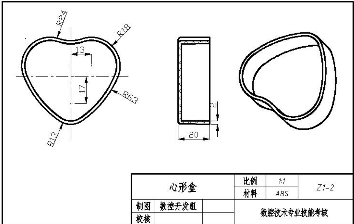
图Z1-2 心形盒
