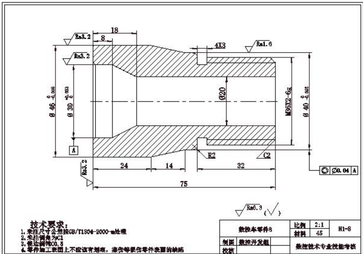
图H1-8 数控车零件8
