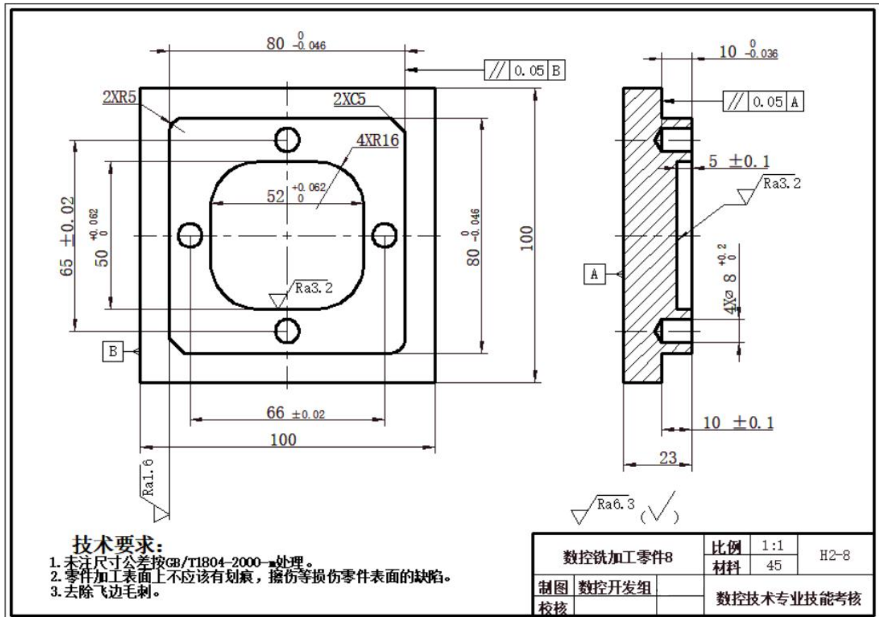
图H2-8 数控铣加工零件8
