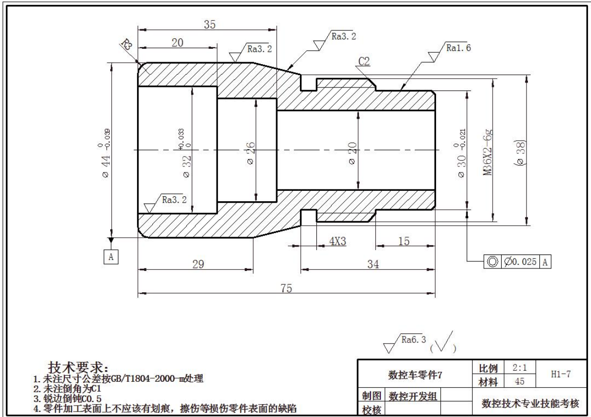
图H1-7 数控车零件7
