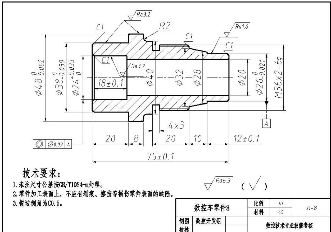
图J1-8 数控车零件8
