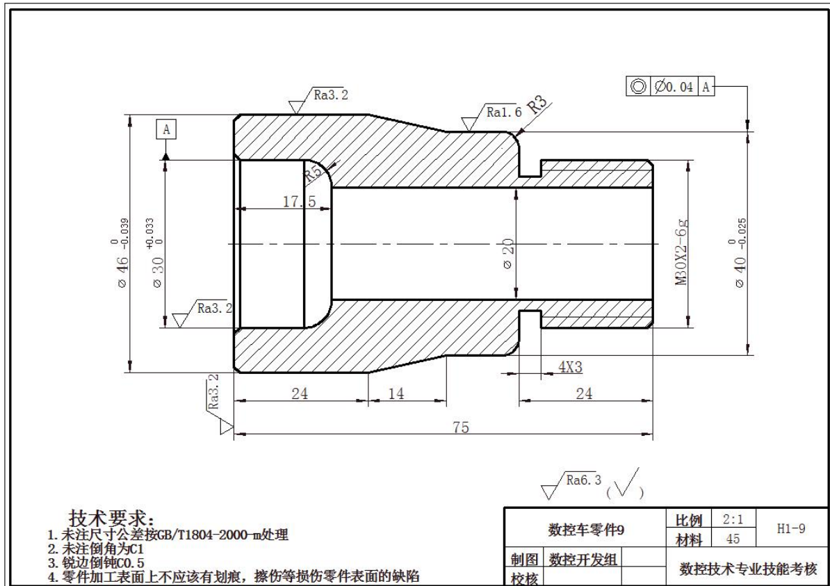
图H1-9 数控车零件9
