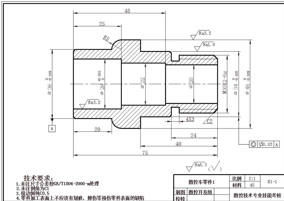
图H1-1 数控车零件1
