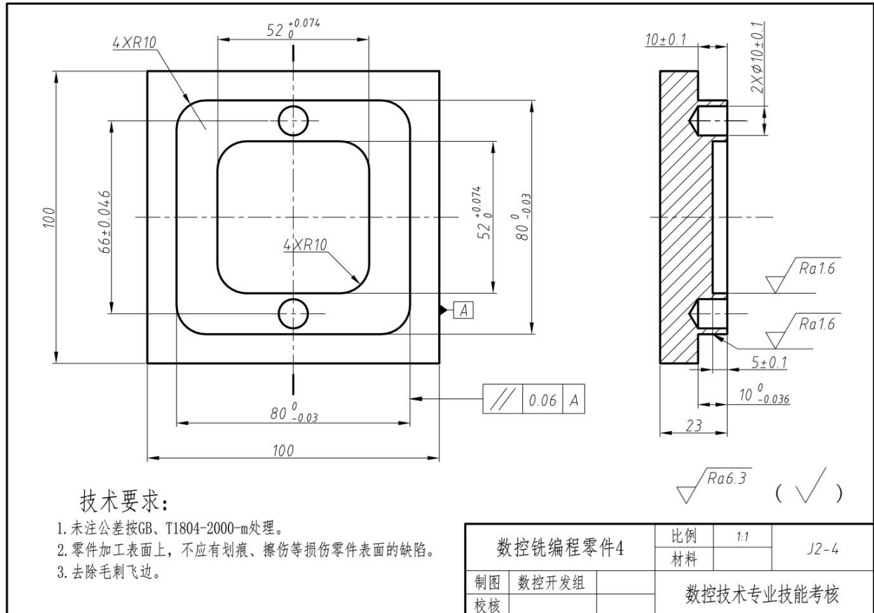
图J2-4 数控铣编程零件4
