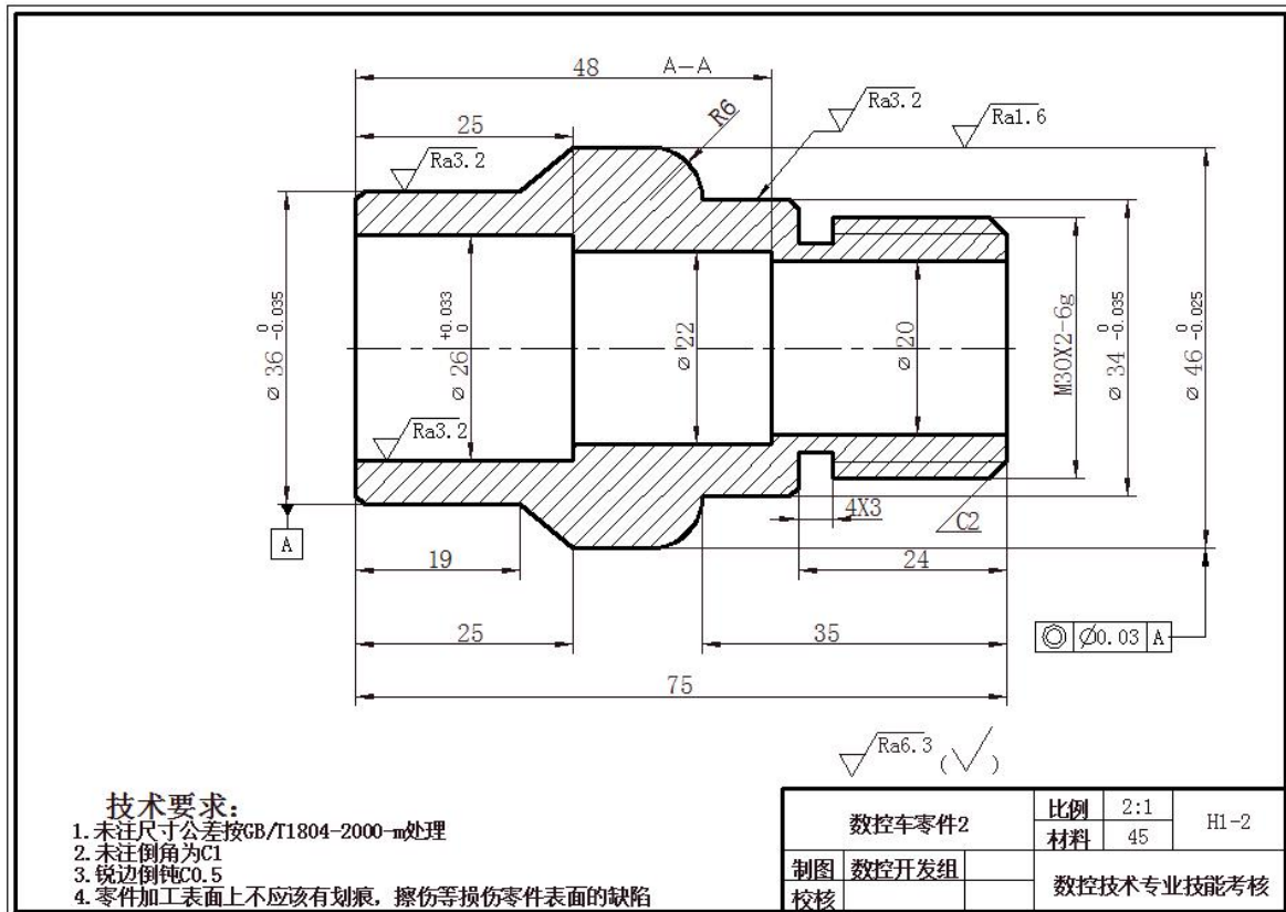
图H1-2 数控车零件2
