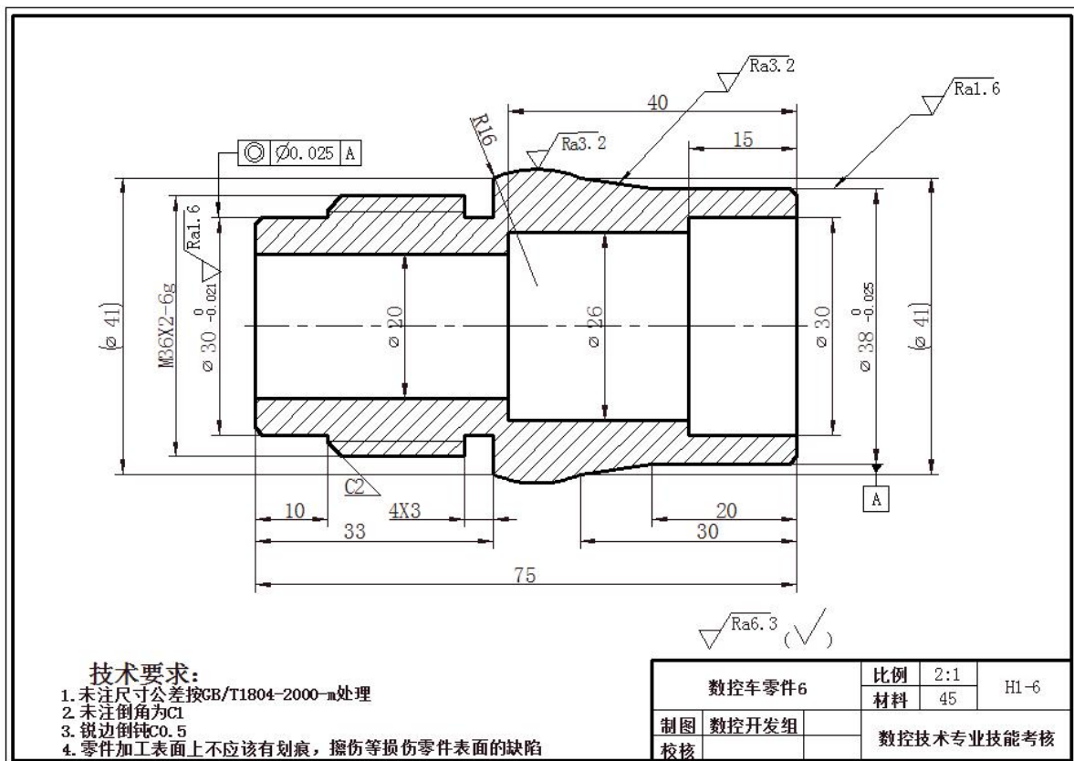
图H1-6 数控车零件6
