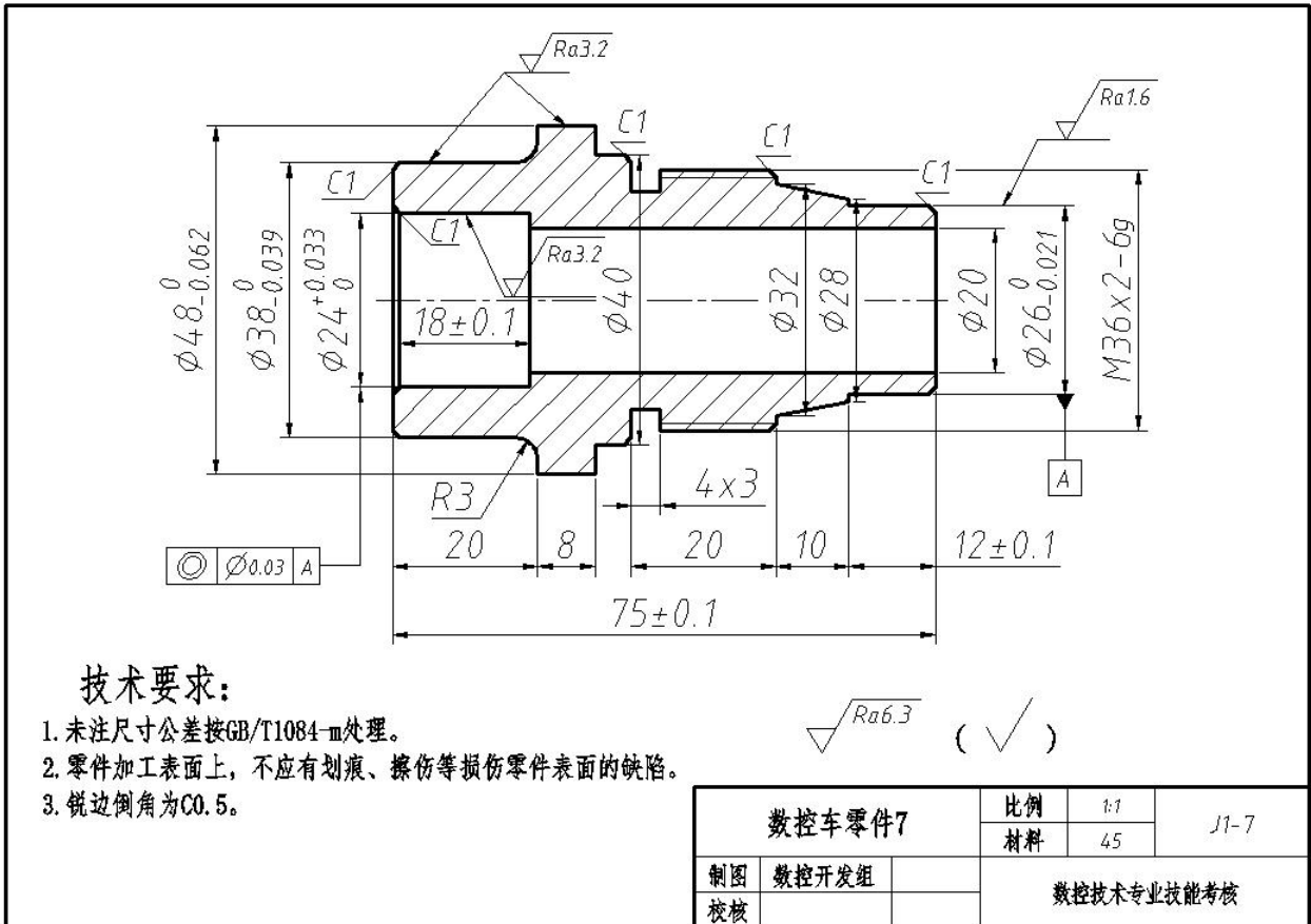
图J1-7 数控车零件7
