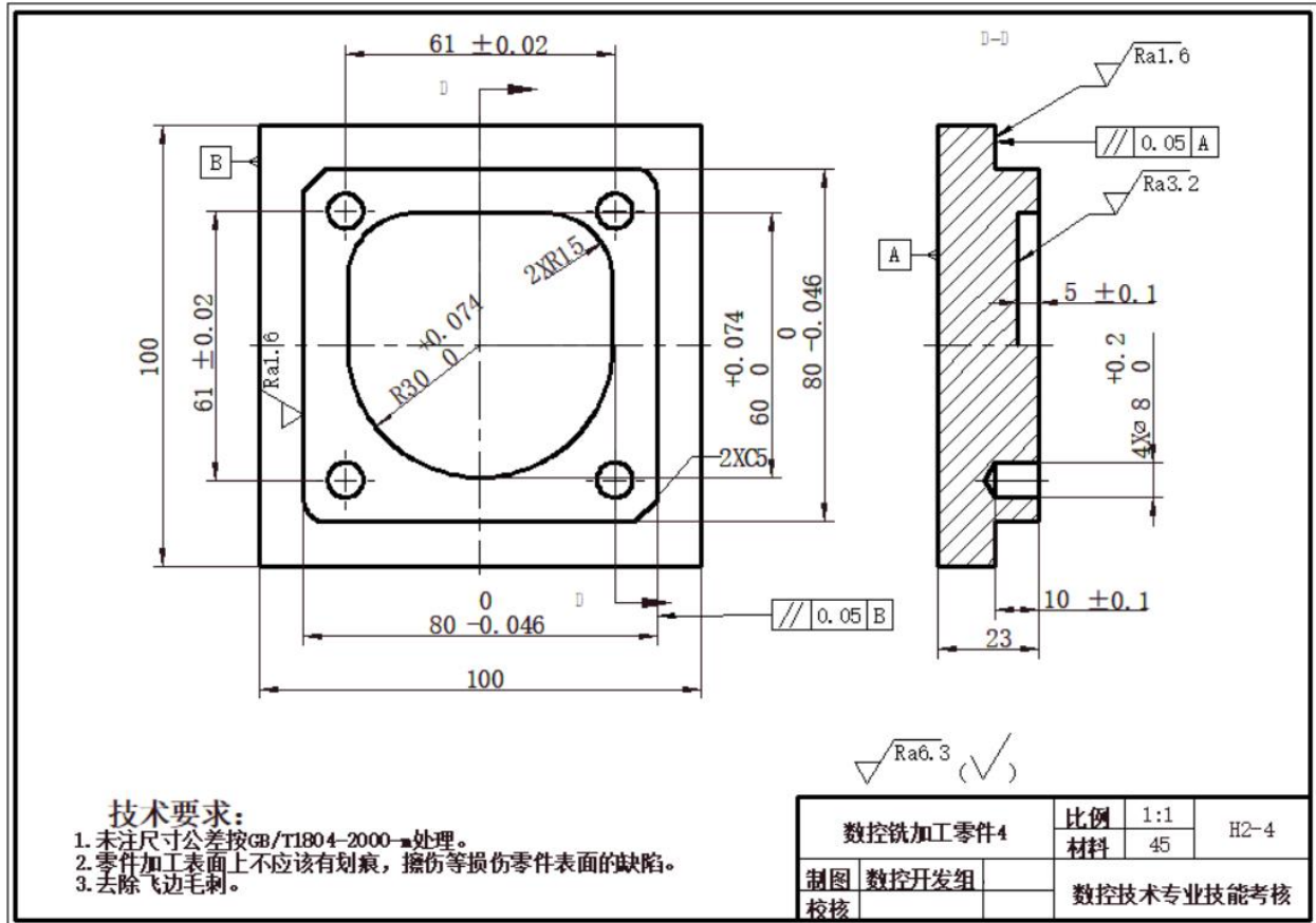
图H2-4 数控铣加工零件4
