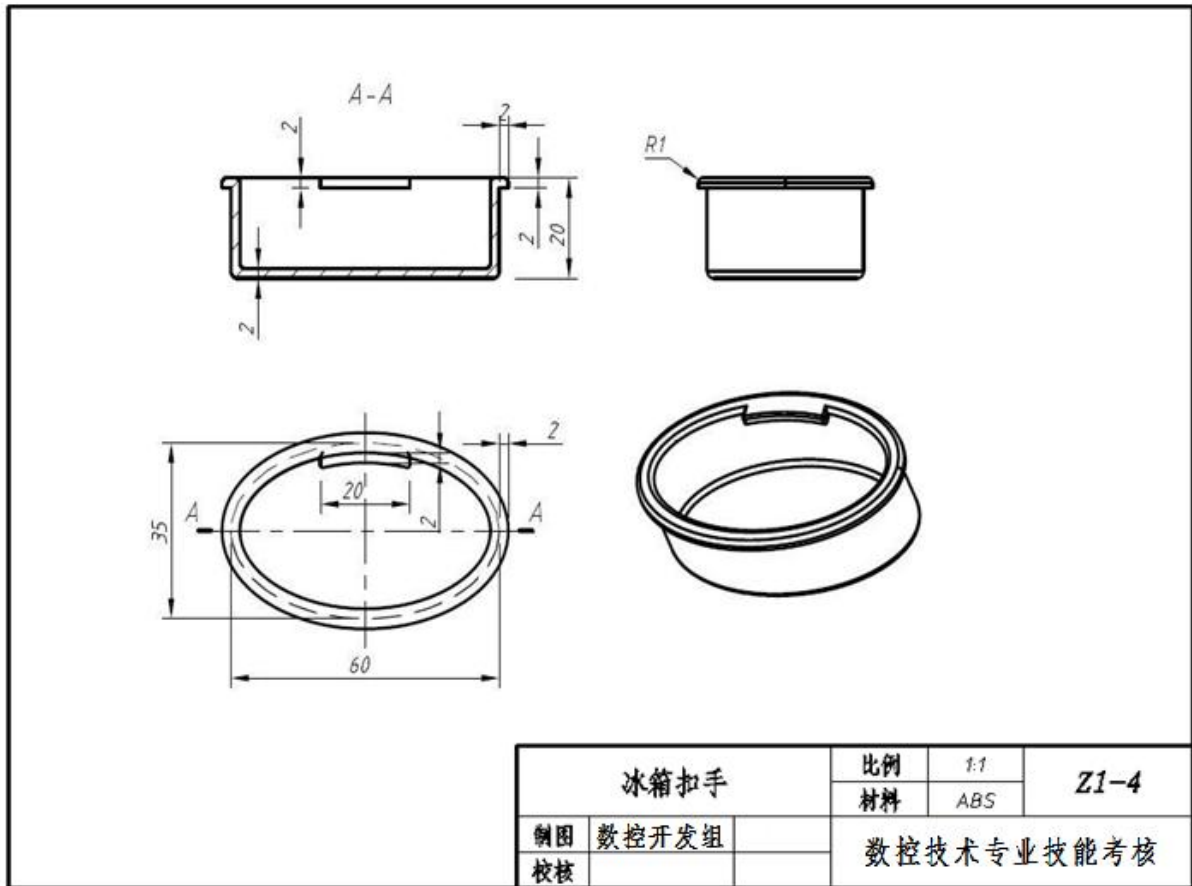
图Z1-4 冰箱扣手
