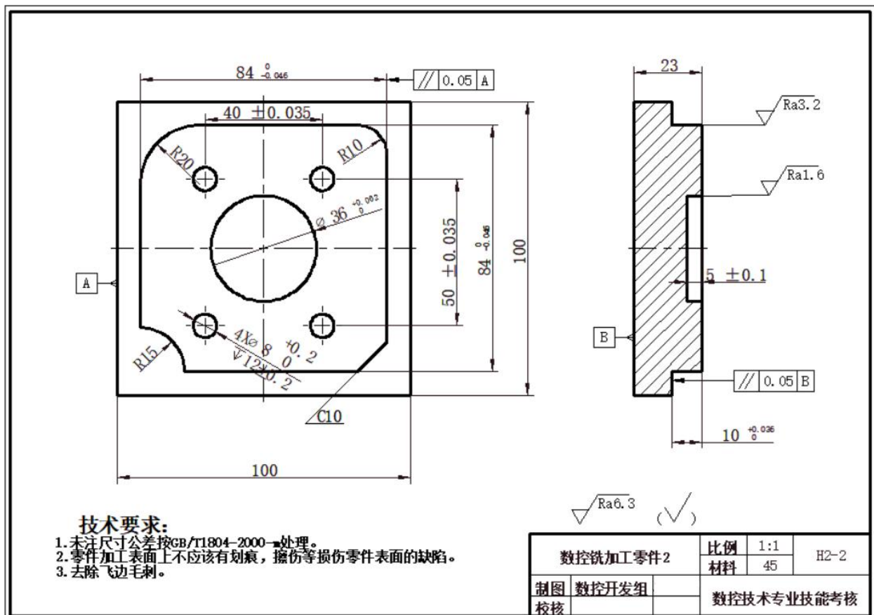
图H2-2 数控铣加工零件2
