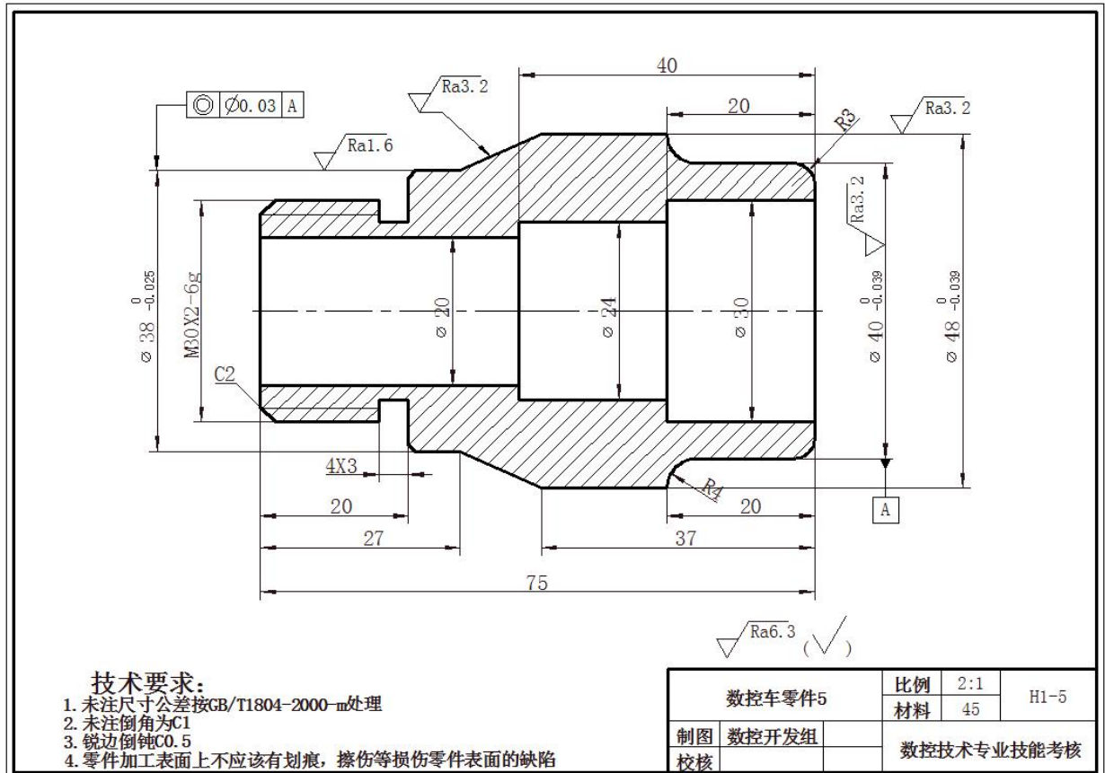
图H1-5 数控车零件5
