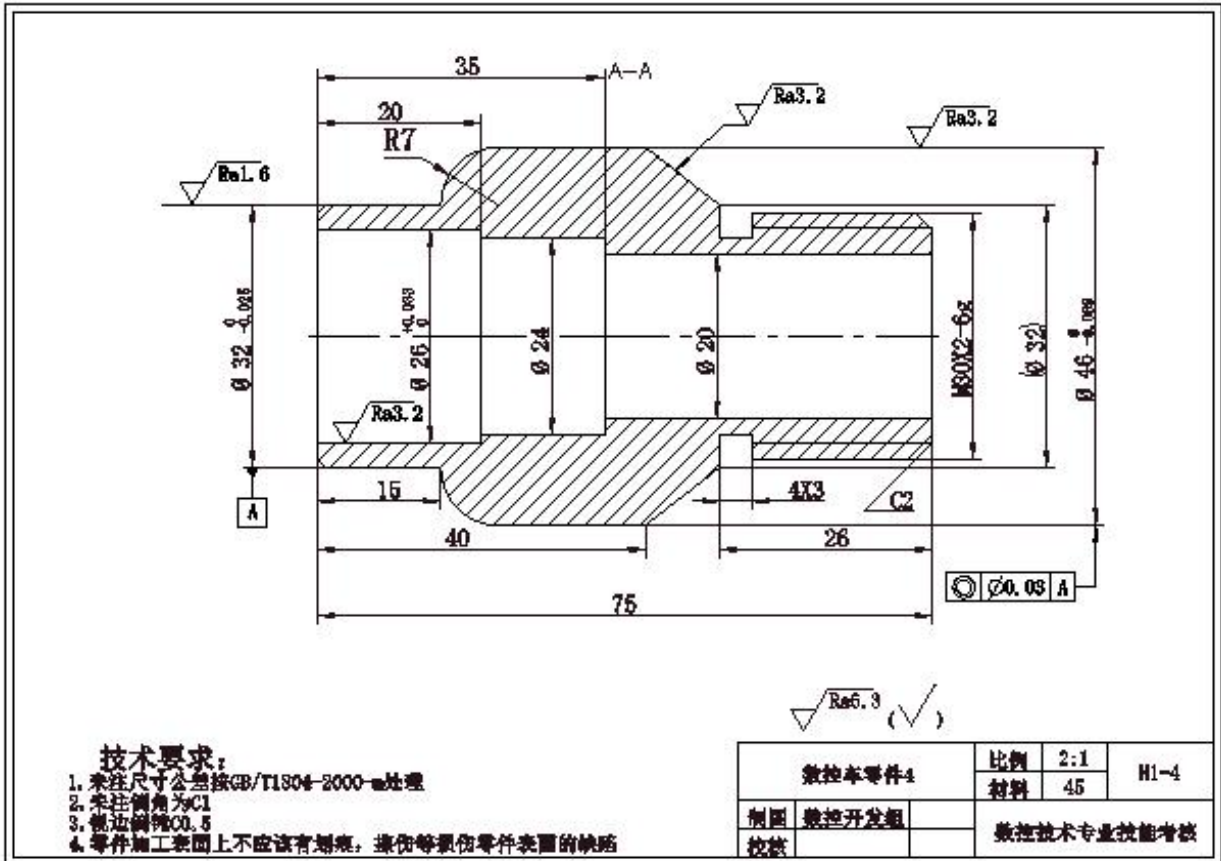
图H1-4 数控车零件4
