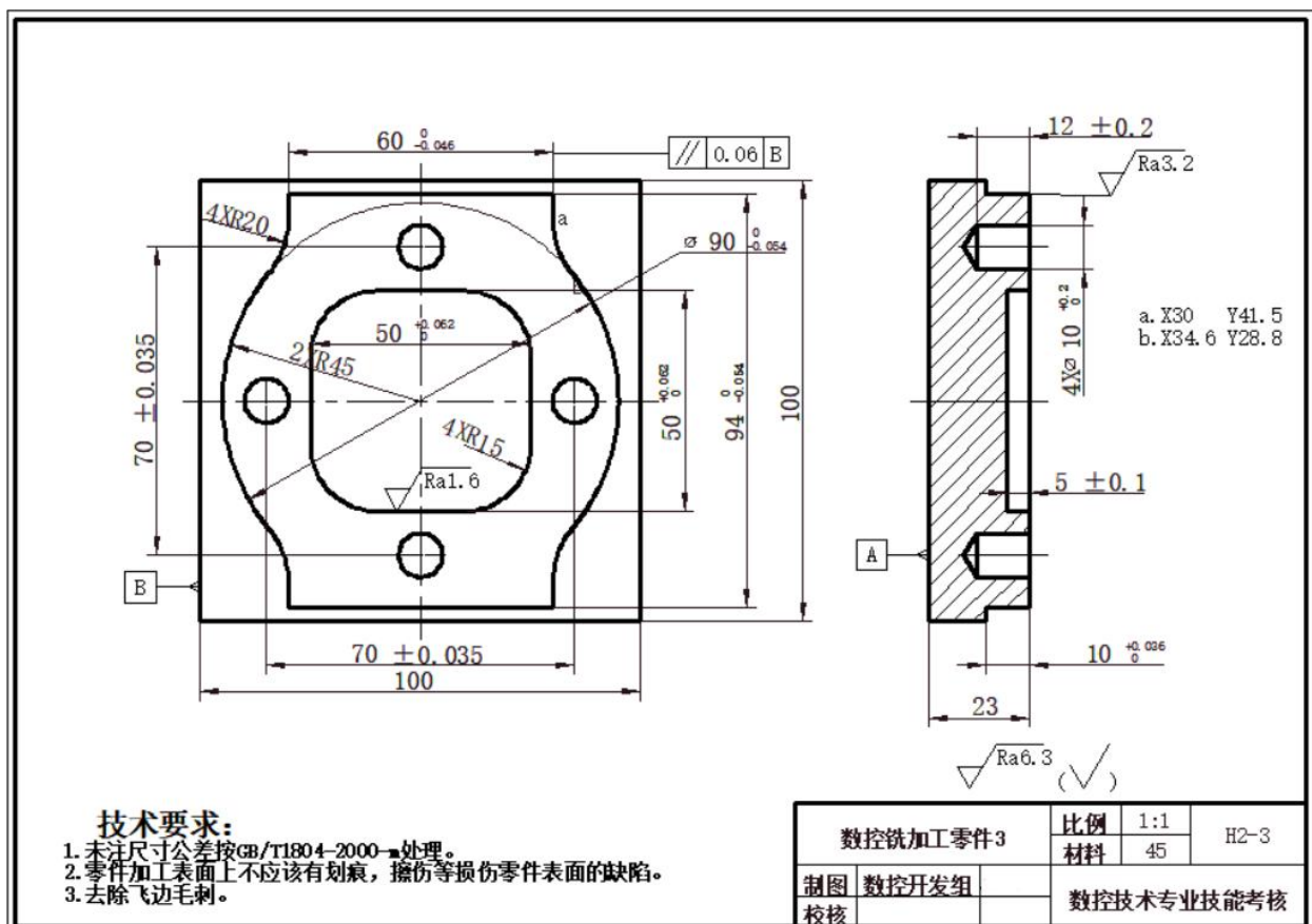
图H2-3 数控铣加工零件3
