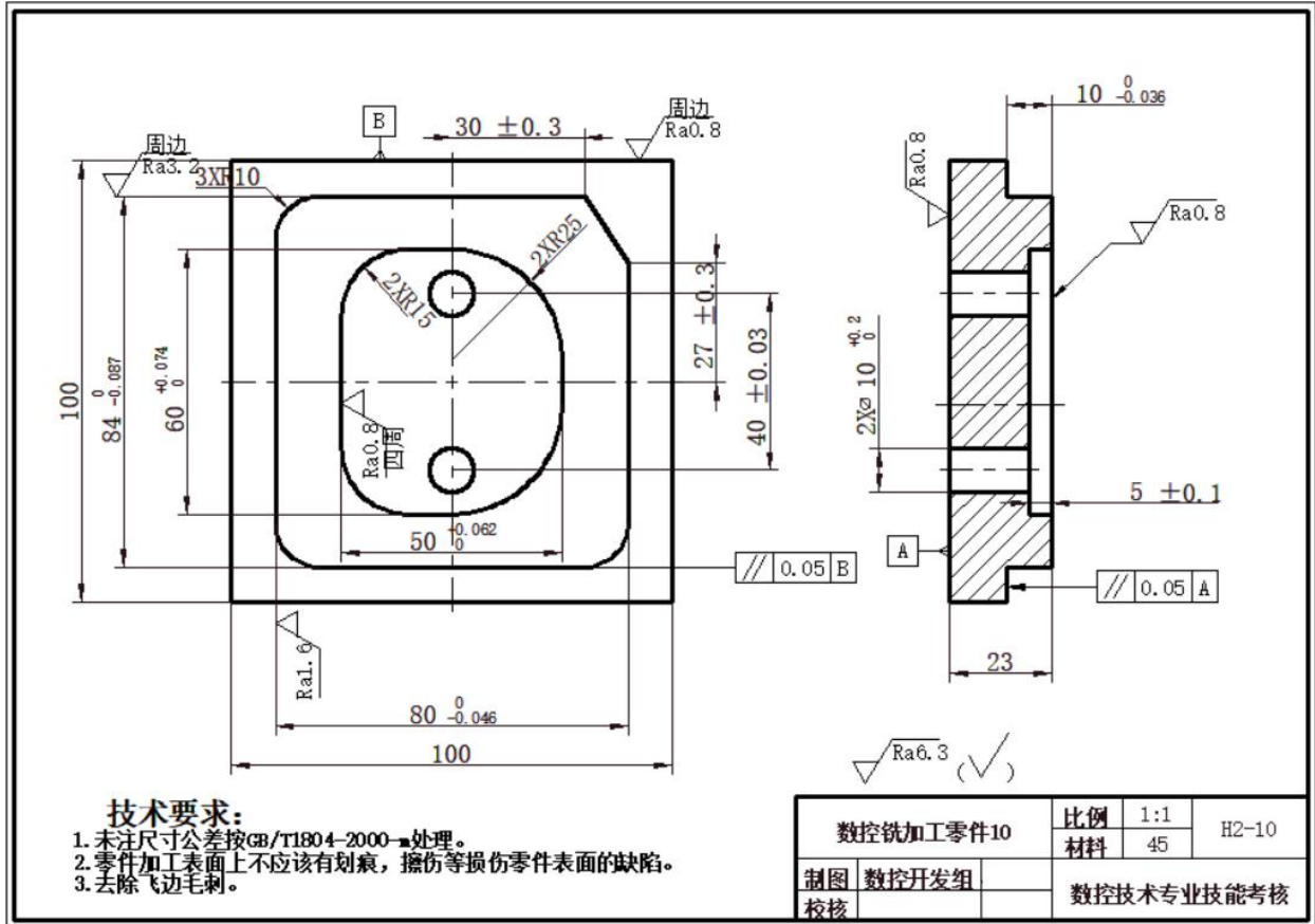
图H2-10 数控铣加工零件10
