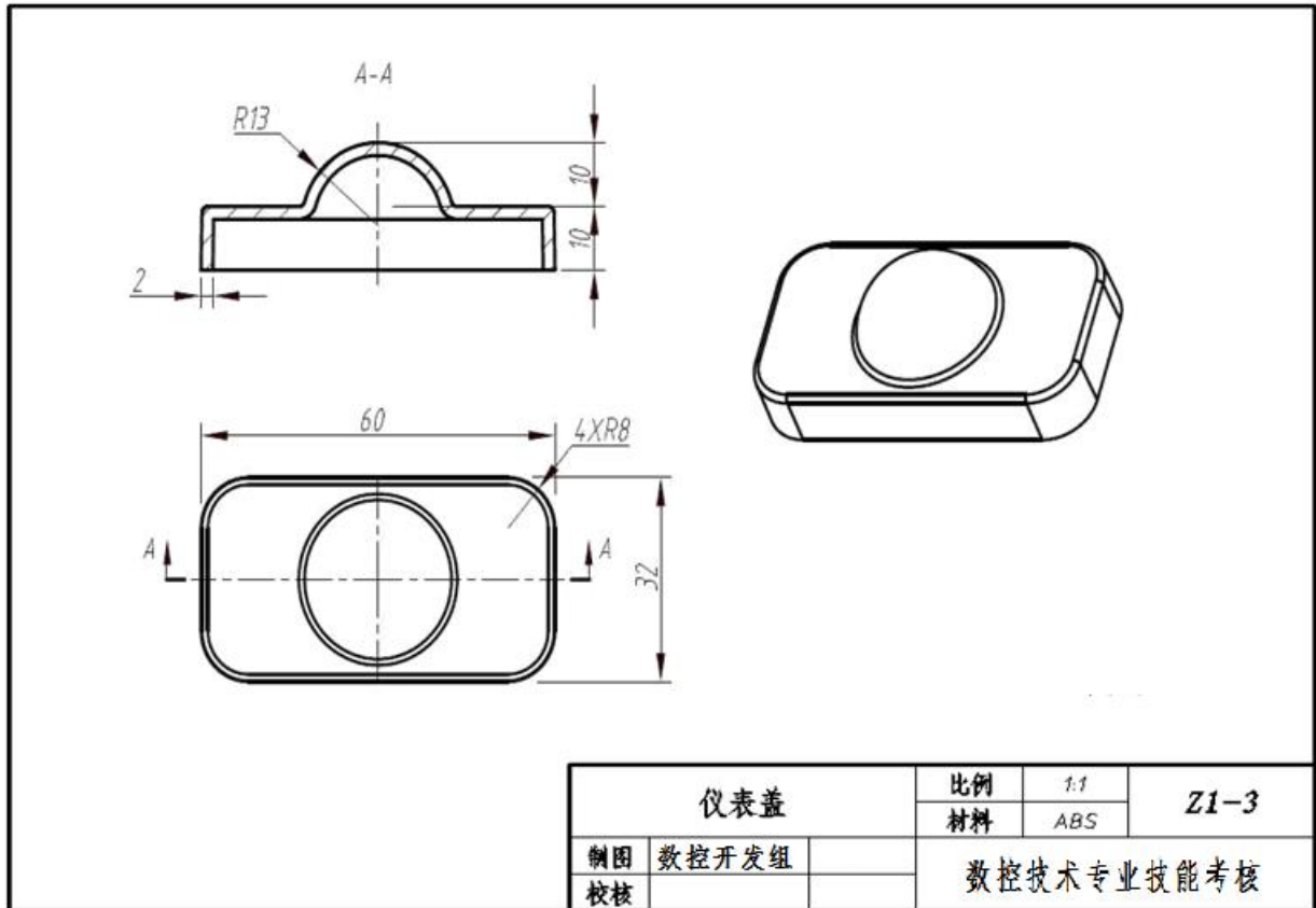
图Z1-3 仪表盖
