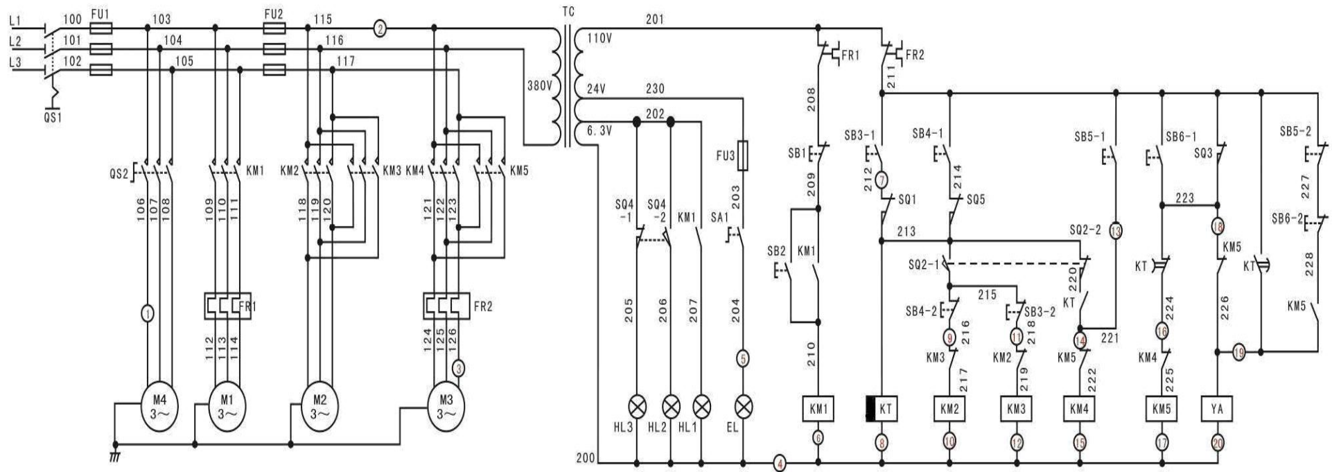
图 2-14 Z3050 摇臂钻床电气控制线路故障图
