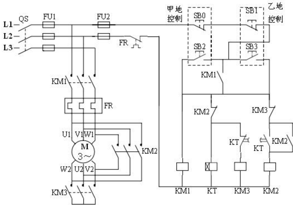
图 3-6 两地控制的电动机 Y—Δ 降压启动控制线路
