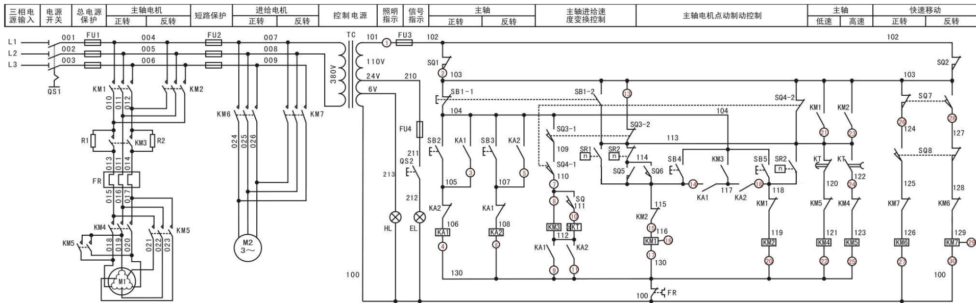
图 2-12 T68 卧式镗床电气控制线路故障图
