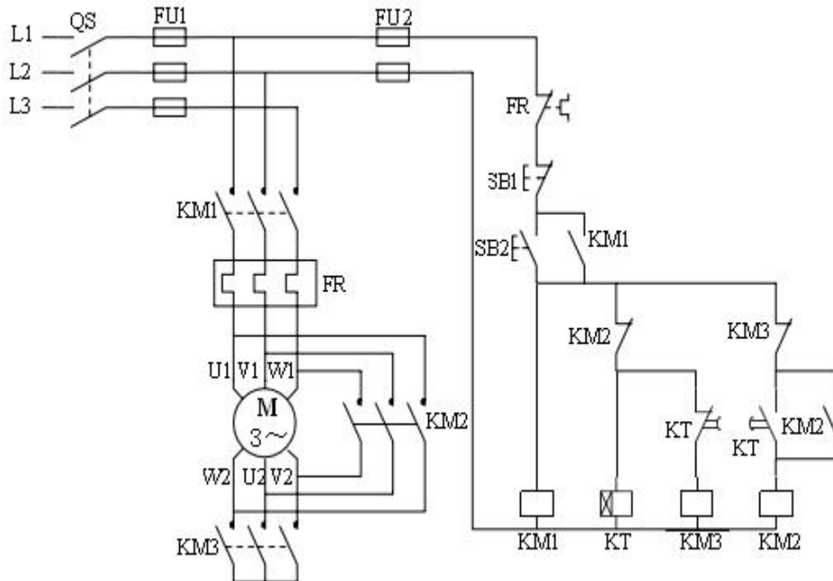
图 3-1 时间继电器控制 Y—△降压启动控制线路图
