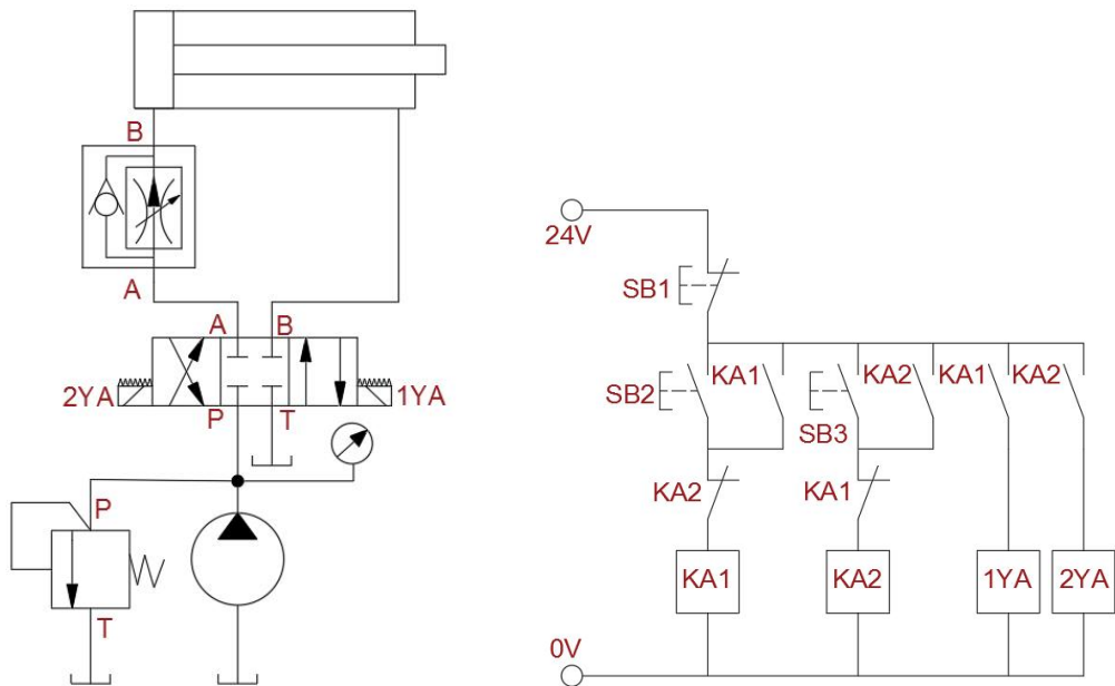
图 2-1-1 进油节流调速回路和电气控制线路图
