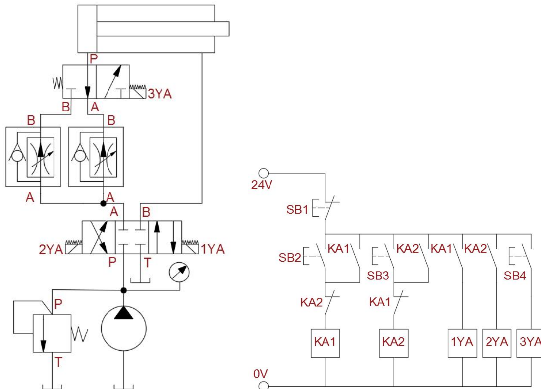
图 2-3 并联调速阀调速回路和电气控制线路图
