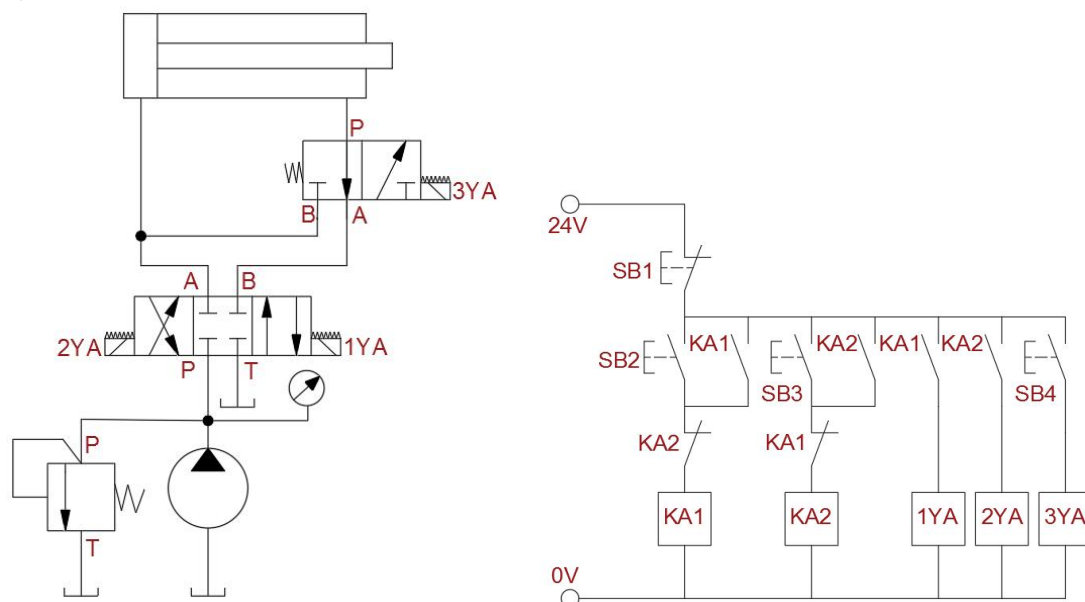
图 2-4 差动连接液压回路和电气控制线路图
