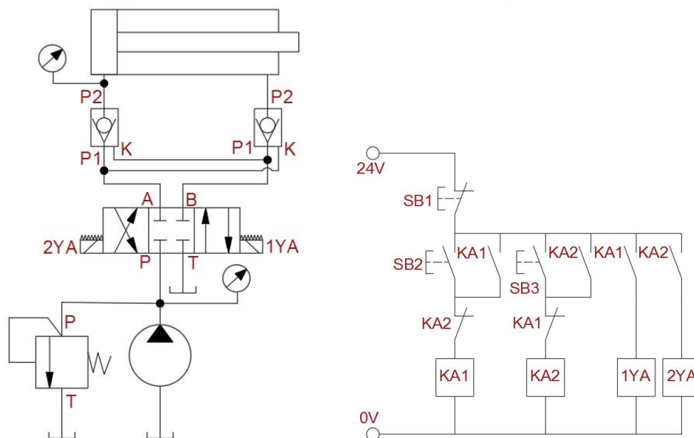
图 2-5 液控单向阀自锁回路和电气控制线路图
