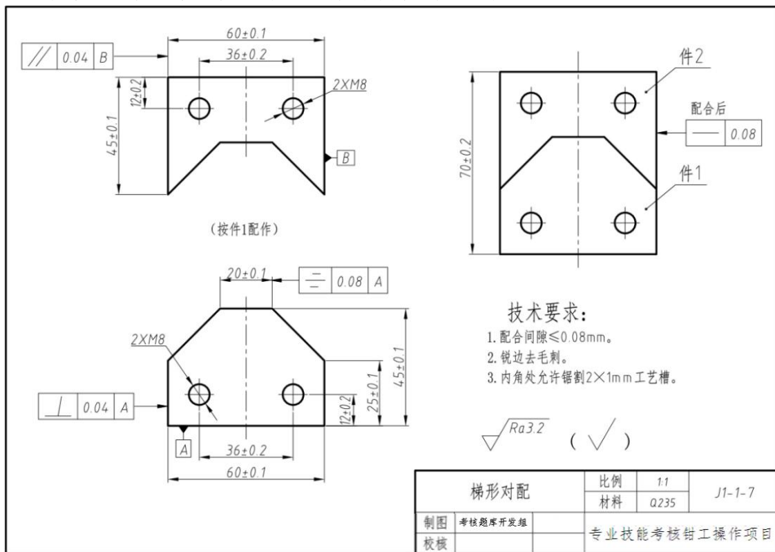
图1-7 梯形对配
