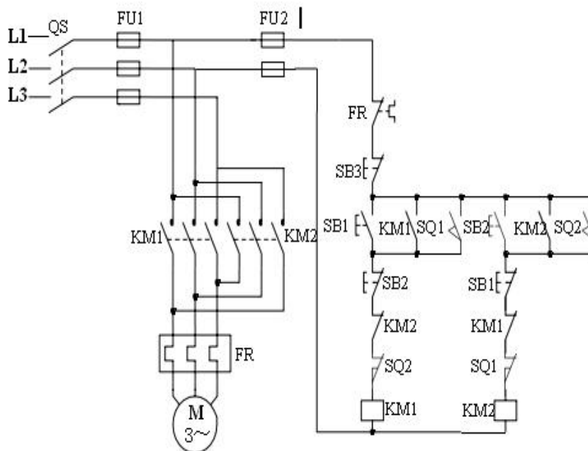
图 3-2 电动机自动往返循环控制线路图
