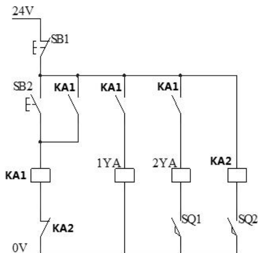
图 3-9 双气缸顺序动作气动回路及电气控制线路图
