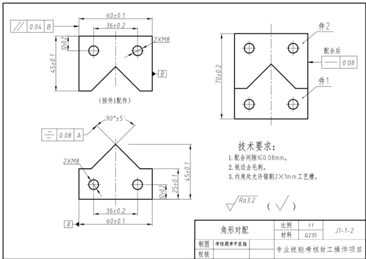
图 1-2 角形对配
