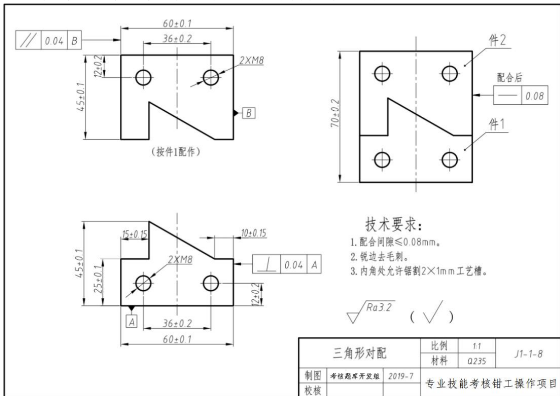
图 1-8 三角形对配
