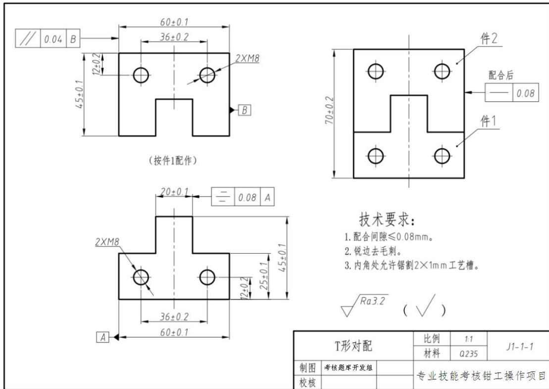
图 1-1 T形对配
