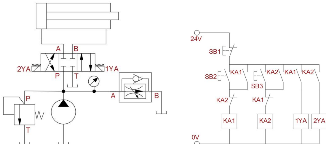
图 2-2 旁油节流调速回路和电气控制线路图
