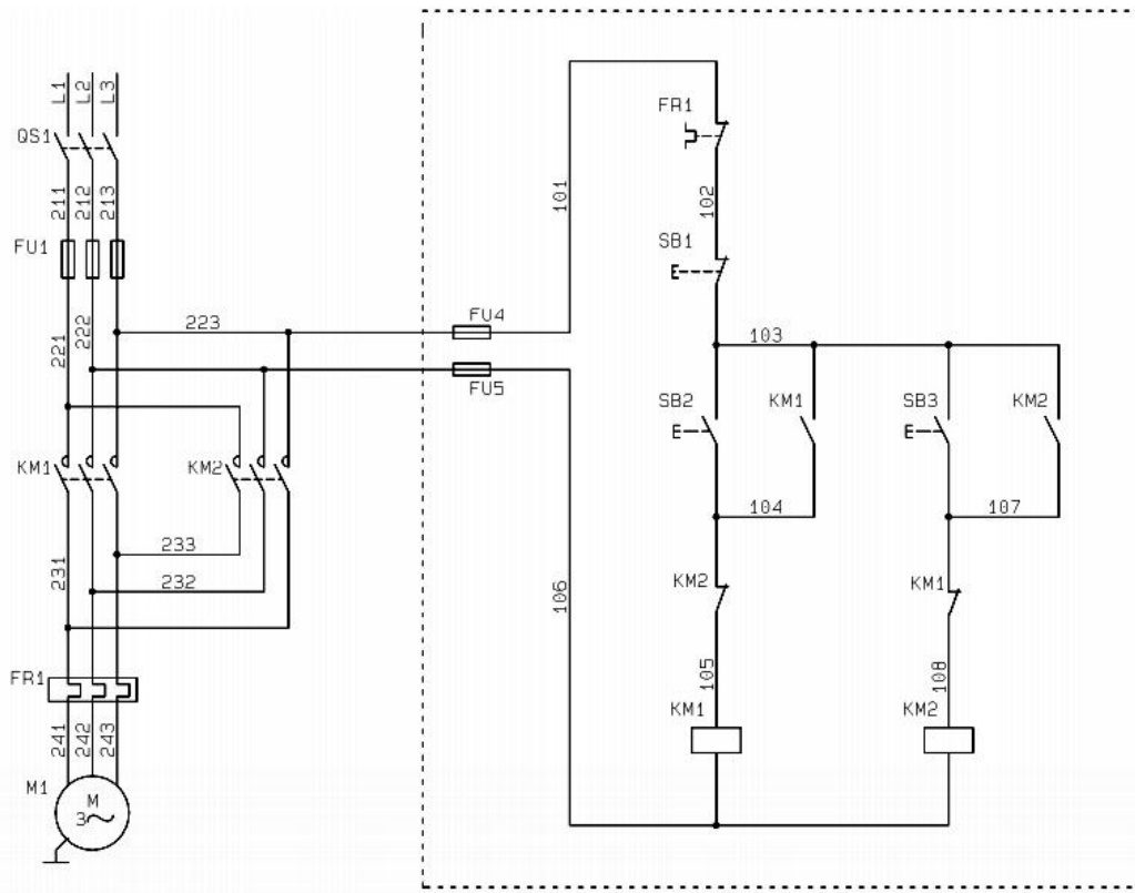
图 1-14 三相异步电动机的正反转控制线路
