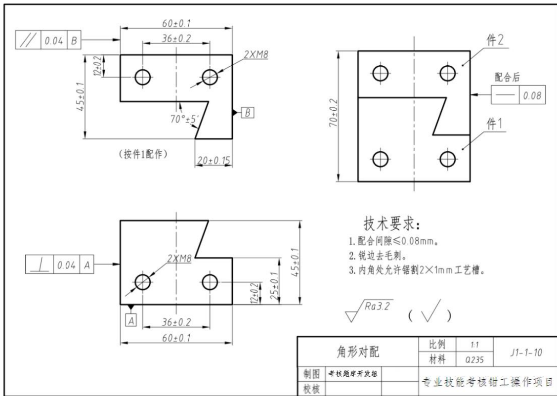
图1-1-10 角形对配
