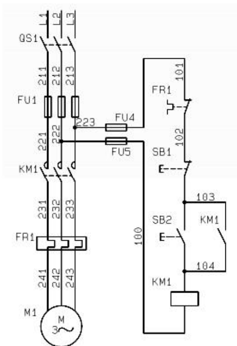
图 1-11 三相异步电动机启动停止线路
