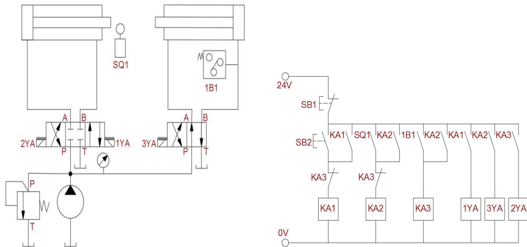
图 2-9 压力继电器和行程开关控制双缸动作顺序回路和电气控制线路图
