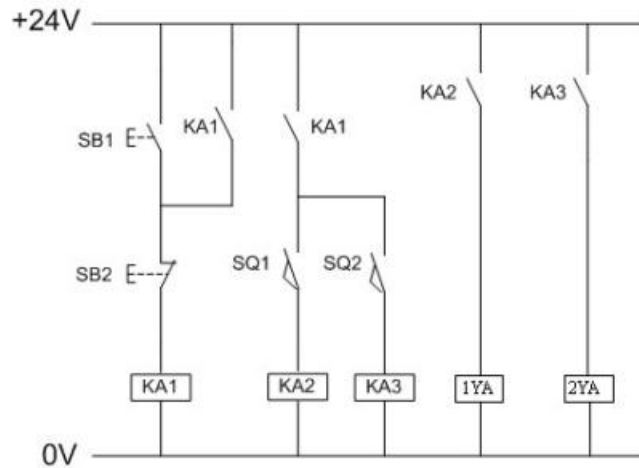
图 3-8 单缸连续自动往返气动回路及电气控制原理图
