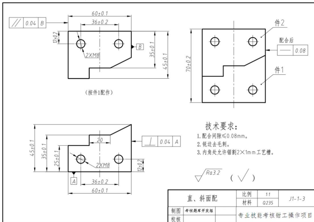
图 1-3 直、斜面配
