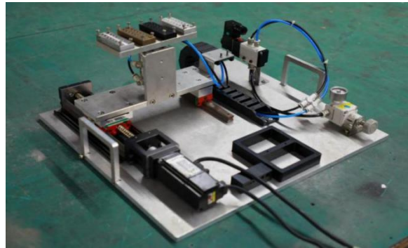
图 16 一种多机构组装的教具
