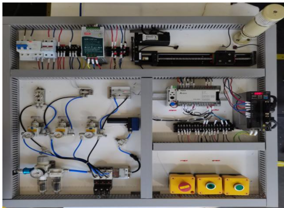
图 17 一种针对 PLC 调试的教具
